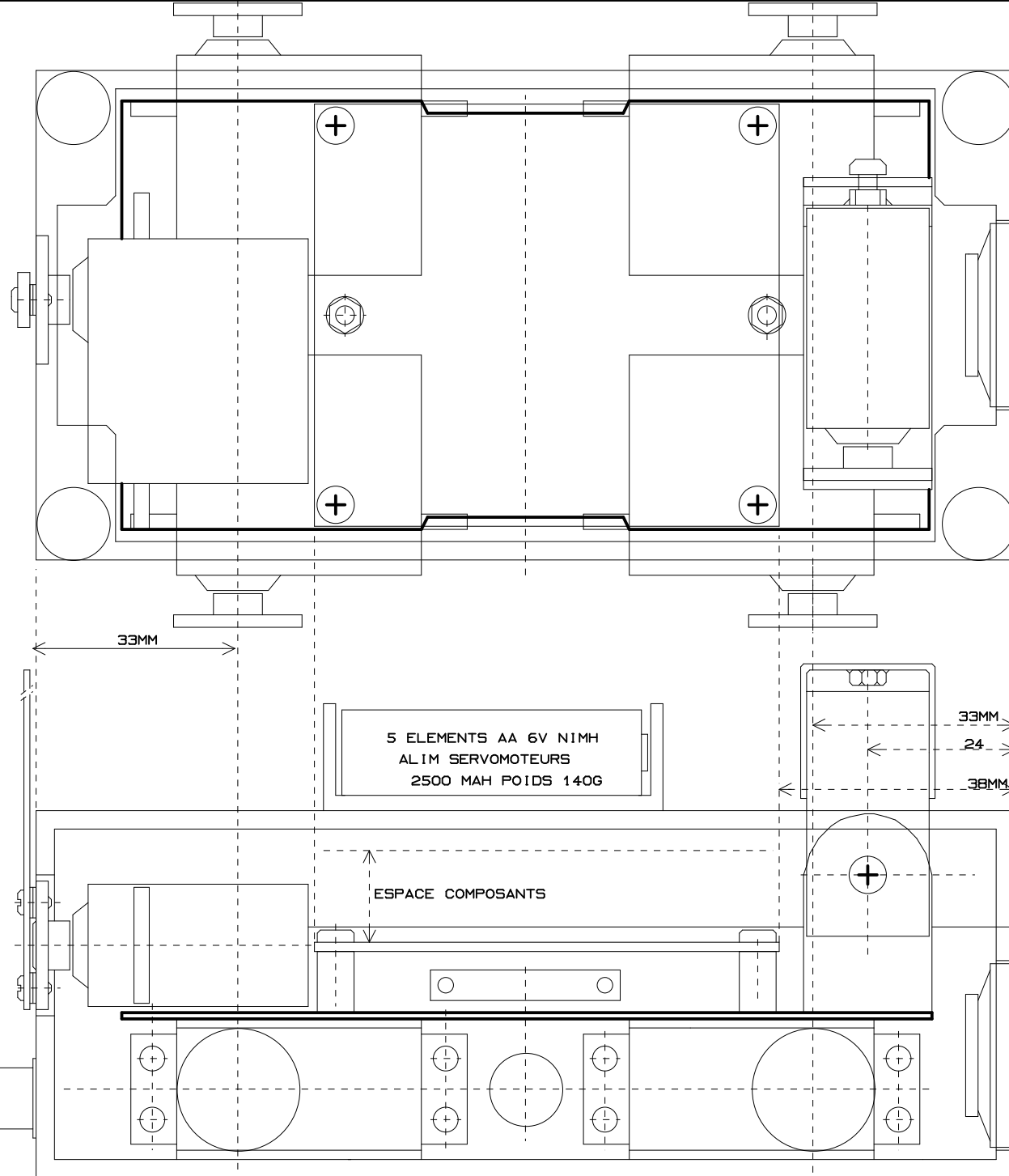
ROBOT CHIEN CORPS VU DE DESSUS
